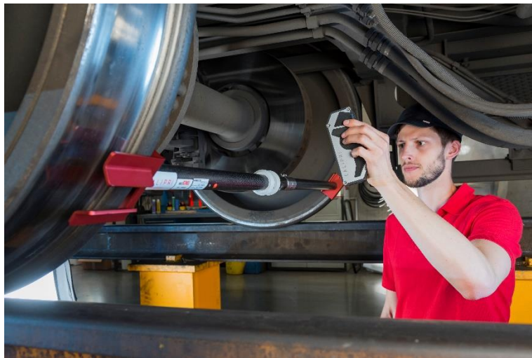
MESSUNG DES RADINNENABSTANDES MIT CALIPRI
